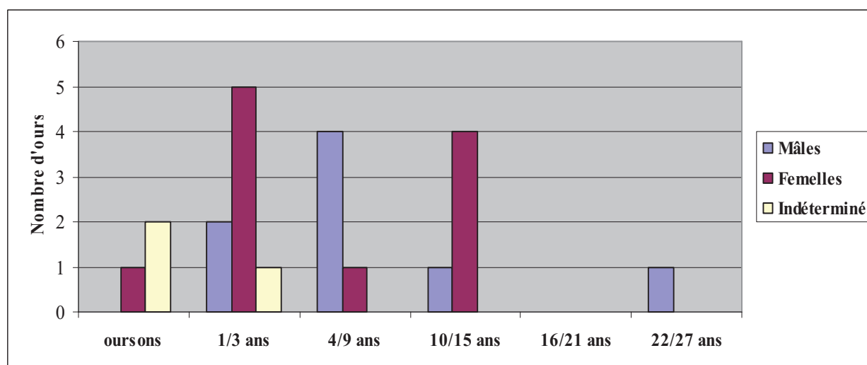
Graphe n° 9. Composition de la population par classe d'âge pour 2012.
