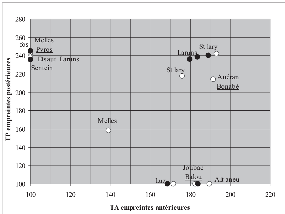
Graphes n° 7. Indices de taille calculés à partir des mesures des empreintes d'ours récoltées dans les Pyrénées françaises en 2012.
