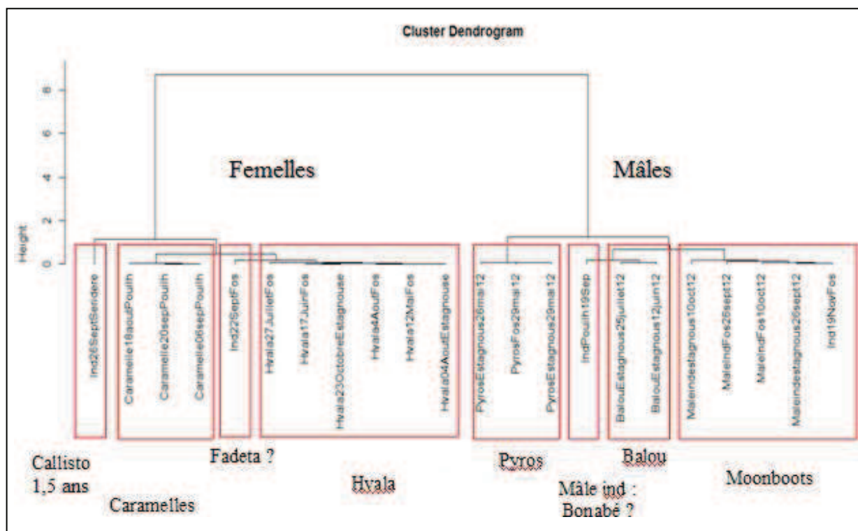
Grappe n° 6. Classification des ours selon leur taille et leur variabilité intra individuelle en fonction des 4 différentes mesures (Cluster dendrogram, Hclust, Ward) (oursons non représentés ici).
