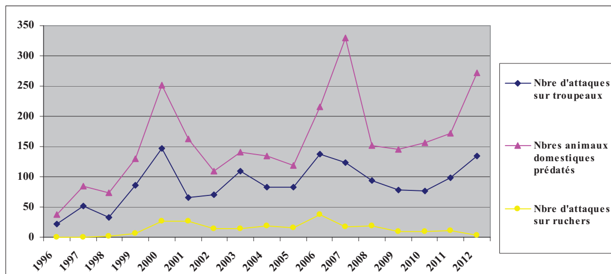
Graphe n° 5. Evolution annuelle du nombre de prédateurs d'ours sur cheptel domestique et sur ruchers dans les Pyrénées françaises depuis 1996.
