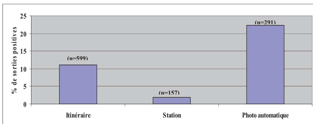
Graphe n° 2. Pourcentage de sorties positives par type de technique : n = nombre de sorties réalisées.
