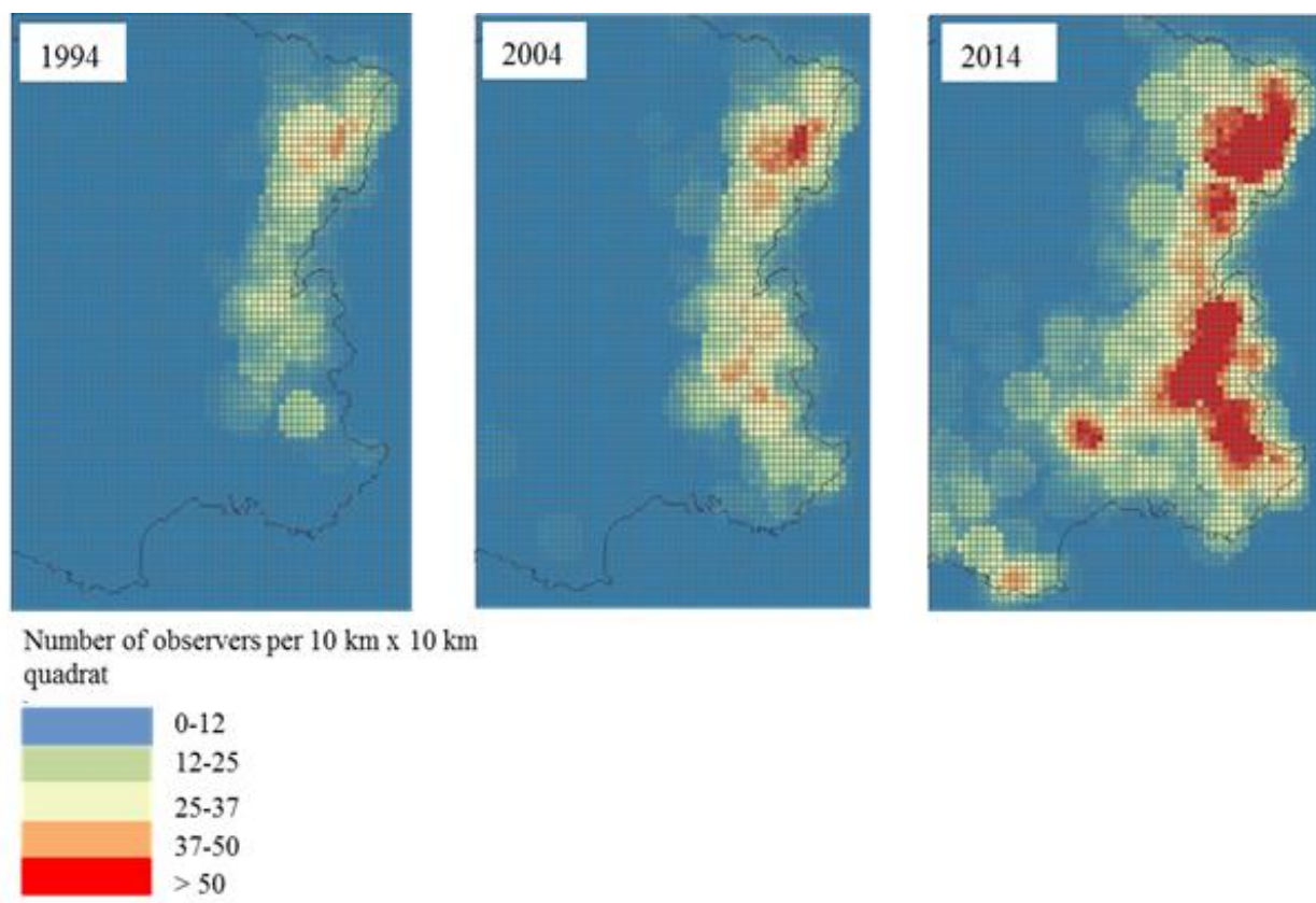
FIGURE 14 CARTES DE L'EFFORT DE PROSPECTION (APPROXIMÉE PAR LE NOMBRE ET LA LOCALISATION DES CORRESPONDANTS DU RESEAU LOUP LYNX / 100 KM 2 ) EN 1994, 2004, ET 2014.
