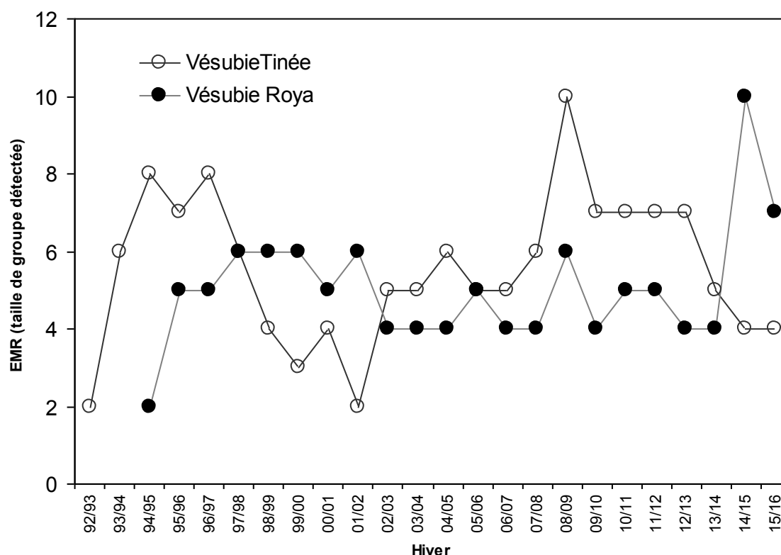
FIGURE 1 VARIATION ANNUELLE DE LA TAILLE DE GROUPE DE 2 MEUTES VOISINES SUR LE MASSIF DU MERCANTOUR, MESUREE PAR L'EMR (NOMBRE MINIMUM D'ANIMAUX SE DEPLAÇANT ENSEMBLE EN PERIODE HIVERNALE), DETECTEE PAR PISTAGE ET OBSERVATIONS VISUELLES. SOURCE : RESEAU LOUP-LYNX.
