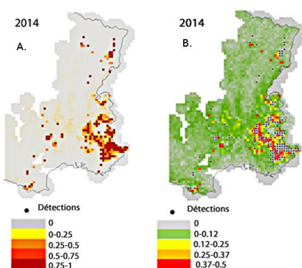
FIGURE 15 CARTES DE L'OCCUPATION ESTIMEE DU LOUP (A) ET DE L'INCERTITUDE ASSOCIEE (B) POUR L'ANNEE 2014. LES POINTS NOIRS SONT LES DETECTIONS REALISEES PAR LE RESEAU DE CORRESPONDANTS EN 2014. TIRE DE LOUVRIER ET AL. 2017.
