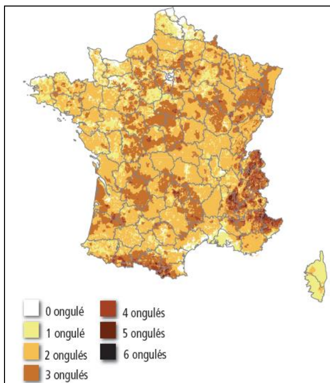
FIGURE 3 CARTE DE PRESENCE DU NOMBRE D'ESPECES DIFFERENTES D'ONGULES : VU LA PLASTICITE ECOLOGIQUE DU LOUP, L'ABONDANCE ET LA DISTRIBUTION DE CES ESPECES NE CONSTITUENT PAS DES FACTEURS PERTINENTS POUR PREDIRE L'EXPANSION DE LA POPULATION DE LOUPS. SOURCE : RESEAU ONGULES SAUVAGES ONCFS/FDC.
