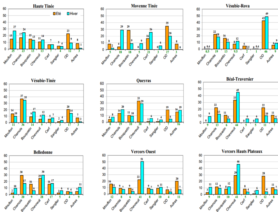
FIGURE 4 RÉGIME ALIMENTAIRE DU LOUP EN FRANCE (N= 1357 FECES), EXPRIME EN NOMBRE D'OCCURRENCES (AXE VERTICAL) DE LA PROIE PRINCIPALE (AXE HORIZONTAL) DIAGNOSTIQUÉES DANS LE NOMBRE DONNÉ D'EXCREMENTS. NB : SUR L'AXE HORIZONTAL, O.D. SIGNIFIE ONGULE DOMESTIQUE. (SOURCE : FLUHR 2008).
