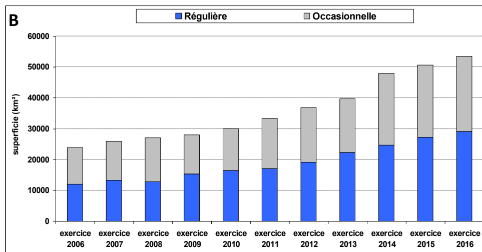
FIGURE 7 A) CARTE DE LA PRESENCE DETECTEE DU LOUP (MAILLES DE 10x10 km) ET B) TENDANCE ANNUELLE OBSERVEE EN FRANCE EN 2016. LA CLASSIFICATION EN PRESENCE REGULIERE OU OCCASIONNELLE EST BASEE SUR UN CRITERE DE NOMBRE MINIMUM D'INDICES ET CONSTATS D'ATTAQUES VALIDES PAR MAILLE ET PAR PERIODE DE DEUX ANNEES BIOLOGIQUES CHEVAUCHANTES (VOIR WWW.ONCFS.GOUV.FR POUR LA METHODE).
