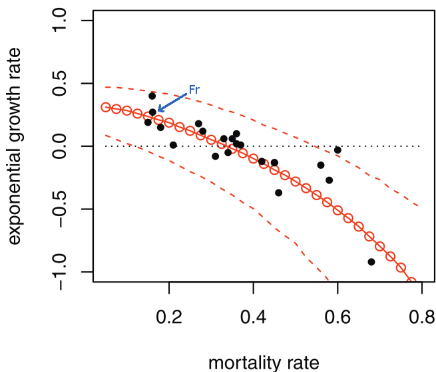
FIGURE 9 MODELISATION (EN ROUGE) DE LA RELATION ENTRE TAUX DE MORTALITE MOYEN (AXE HORIZONTAL) ET CROISSANCE OBTENUE (AXE VERTICAL) D'UNE POPULATION DE LOUPS SIMPLIFIEE EN DEUX CLASSES SOCIALES (ADULTES REPRODUCTEURS ET DISPERSEURS). CE MODELE EST ENSUITE CONTRAINT A S'AJUSTER AUX POINTS NOIRS REPRESENTANT LES DONNEES DE DIFFERENTES POPULATIONS DE LOUPS, INCLUANT LA DONNEE DE LA POPULATION FRANÇAISE OBSERVEE POUR LA PERIODE 1995-2003 (FLECHE BLEUE). L'AJUSTEMENT DU MODELE AUX DONNEES DE TERRAIN ETANT STATISTIQUEMENT BON, IL PEUT ETRE UTILISE POUR PREDIRE QU'EN MOYENNE, UN SEUIL DE MORTALITE DE 34% ENTRAINE LA POPULATION SUR UNE PHASE DECROISSANTE (FIGURE ISSUE DE MARESCOT ET AL. 2012).
