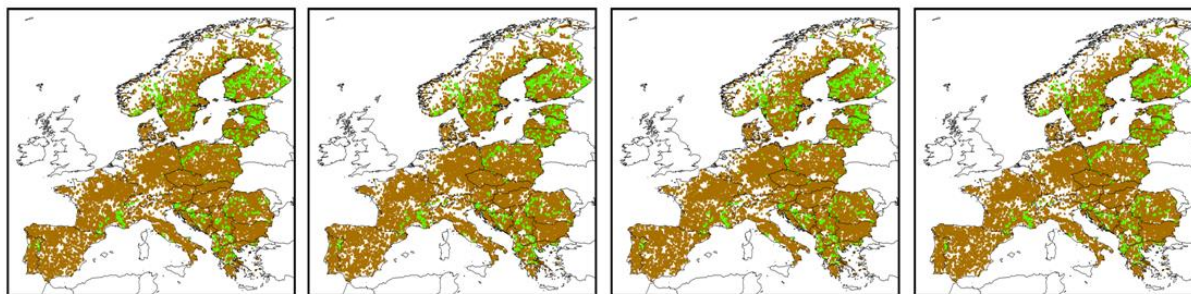
FIGURE 17. PROJECTION D'UNE DISTRIBUTION PREVISIONNELLE MACRO-ECOLOGIQUE DU LOUP EN EUROPE A L'HORIZON 2040 SOUS DIFFERENTS SCENARIOS DE CHANGEMENT DES HABITATS ET DE LEUR EXPLOITATION PAR L'HOMME (DE GAUCHE A DROITE : GRADIENT DE CROISSANCE ECONOMIQUE DE FORT A MODERE). TIRE DE MILANESI ET AL. (2016). EN VERT : SUPERPOSITION AVEC LA PRESENCE DEJA DETECTEE TIREE DE CHAPRON ET AL. 2014. EN MARRON : PRESENCE PREDITE.
