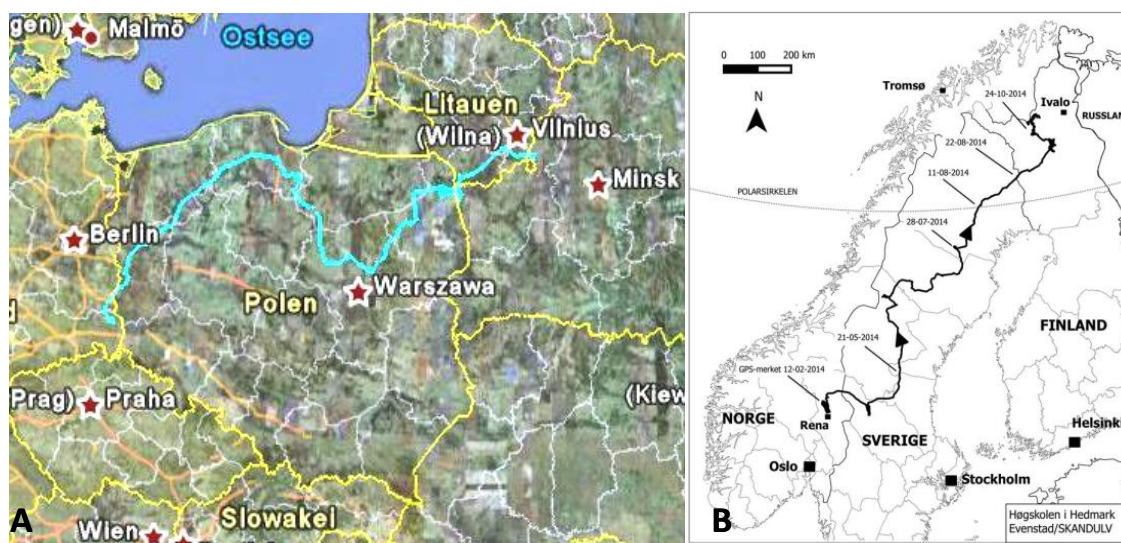
FIGURE 2 EXEMPLES DE DISTANCES PARCOURUES PAR LE LOUP EN PHASE DE DISPERSION* (SUIVI GPS/GSM) ; A) DISTANCE EQUIVALANT A 800 KM EN LIGNE DROITE EN ALLEMAGNE ENTRE LE 23/04 ET LE 12/10/2009 (I. REINHARD, LUPUS CONSULTING). B) DISTANCE EQUIVALANT A 1200 KM EN LIGNE DROITE EN SUEDE ENTRE LE 12/02 ET LE 24/10/2014 (C. MILLERET, SKANDULV).
