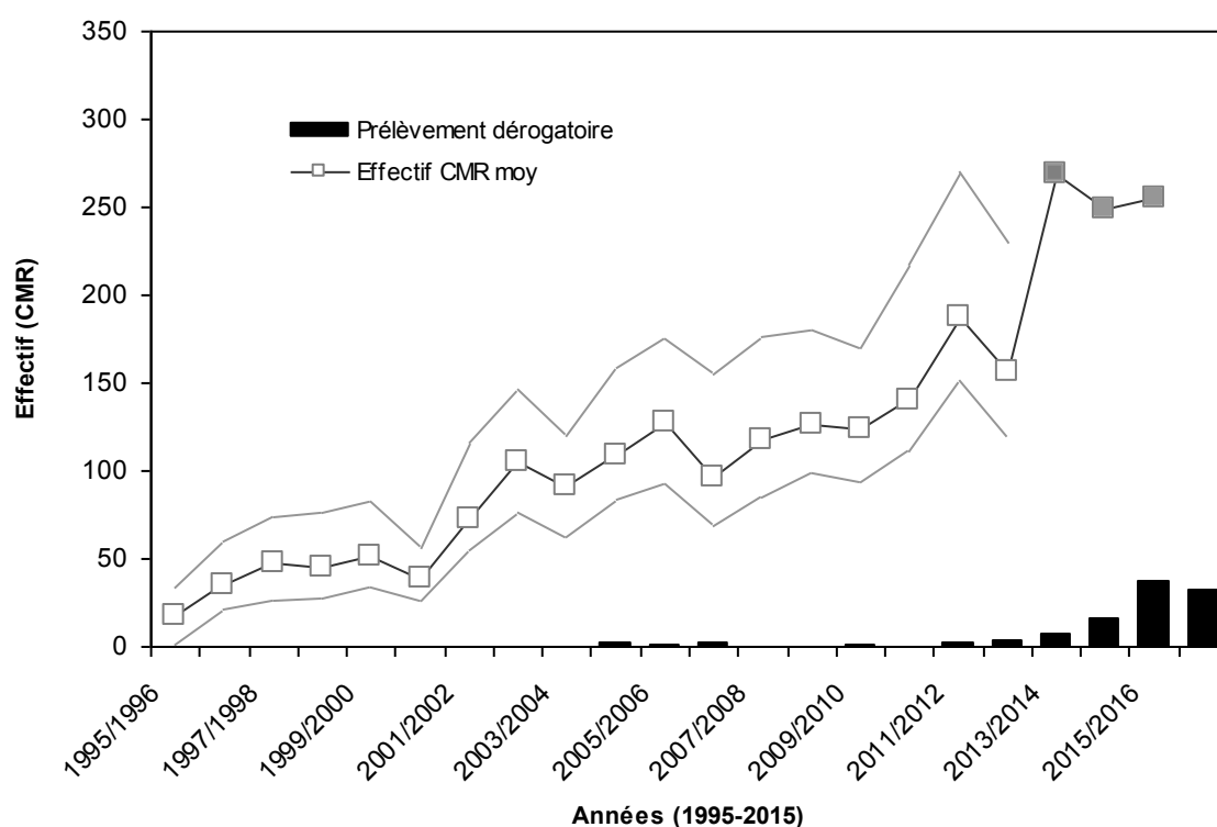
FIGURE 10 ESTIMATION DES EFFECTIFS DE LA POPULATION DE LOUPS EN FRANCE SUR LA BASE DES MODELES DE CAPTURE-MARQUAGE-RECAPTURE (CMR) APPLIQUES AUX PROFILS GENETIQUES ETABLIS PAR LE SUIVI BIOMOLECULAIRE DES EXCREMENTS, POILS, URINES, SANG OU TISSUS (VOIR CUBAYNES ET AL. 2010 POUR LA METHODE). LE MODELE EST REAJUSTE SUR LA BASE DES DONNEES GENETIQUES DISPONIBLES (1995-2013 ; CARRE BLANC). LES POINTS DE 2014 A 2016 (CARRES GRIS) SONT PROJETES SUR LA BASE DE LA RELATION CALIBREE DE LA CMR EN FONCTION DE L'EFFECTIF MINIMUM DENOMBRE DANS LES ZPP (INDICATEUR EMR). CETTE RELATION PERMET EN EFFET DE PASSER D'UN EFFECTIF MINIMUM RETENU* SUR SEULES ZPP A UN EFFECTIF TOTAL SUR TOUTE L'AIRE DE PRESENCE. L'HISTOGRAMME INDIQUE LE NOMBRE D'ANIMAUX PRELEVES DANS LE CADRE DES TIRS DEROGATOIRES ACCORDES.
