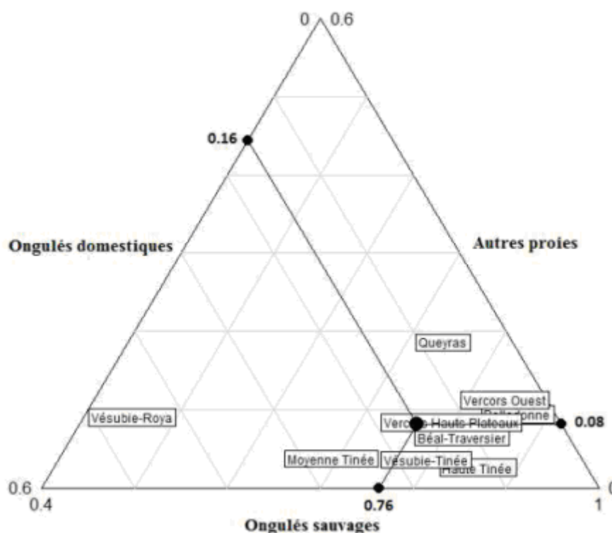
FIGURE 5 PROPORTION DES ONGULÉS DOMESTIQUES, DES ONGULÉS SAUVAGES ET AUTRES PROIES CONSOMMÉES PAR LE LOUP SUR 9 MEUTES FRANÇAISES À PARTIR DE L'ANALYSE DE 1357 EXCREMENTS ANALYSÉS (EXTRAIT DE FLUHR 2008).
