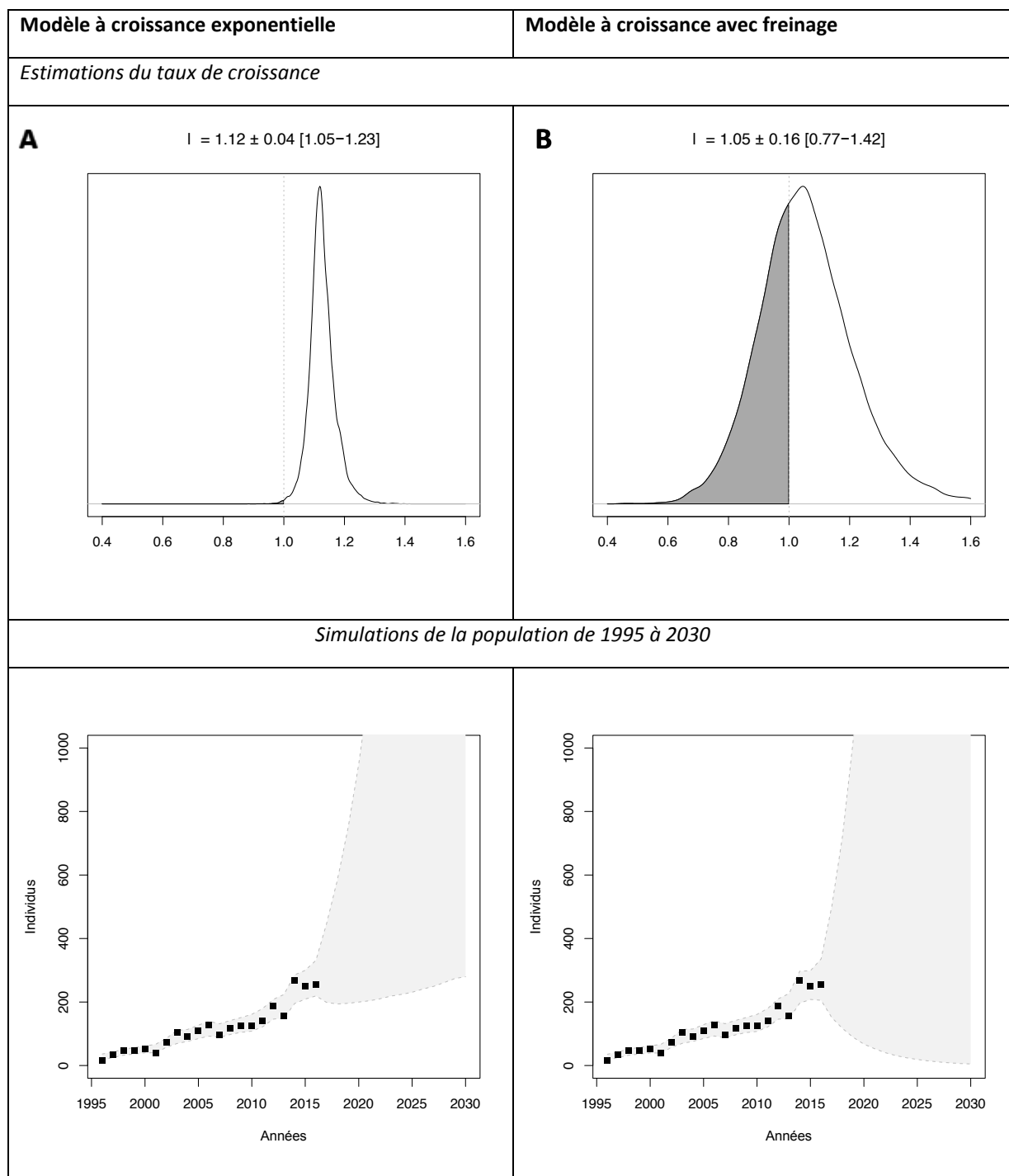
FIGURE 13 AJUSTEMENT DES MODELES DE CROISSANCE DE LA POPULATION DE LOUPS POUR A) (COLONNE GAUCHE) UNE CROISSANCE EXPONENTIELLE MONOTONE ET B) (COLONNE DROITE) UNE CROISSANCE AVEC FREINAGE POUR PRENDRE EN COMPTE LA DYNAMIQUE RECENTE DE LA POPULATION TELLE QUE PRESENTIEE SUR LES 3 DERNIERES ANNEES DE LA SERIE DE DONNEES. PREMIERE LIGNE : DISTRIBUTION DU TAUX DE CROISSANCE* ESTIME PAR LE MODELE. LE PIC DE LA COURBE CORRESPOND A LA VALEUR DU TAUX DE CROISSANCE* (SUR L'AXE HORIZONTAL) QUI EST LA PLUS VRAISEMBLABLE, LA ZONE GRISEE FONCEE INDIQUE LA PROBABILITE QUE LA POPULATION DECROISSE. DEUXIEME LIGNE : SIMULATIONS DE LA POPULATION DE 1995 A 2030. DE 1995 A 2016, LES MODELES SONT AJUSTES AUX DONNEES (CARRS NOIRS). DE 2017 A 2030, LES MODELES PROJETENT LA POPULATION AVEC LES PARAMETRES ISSUS DE L'AJUSTEMENT. LES ZONES GRISEES MONTRENT LES INTERVALLES DE CONFIANCE A 95%.
