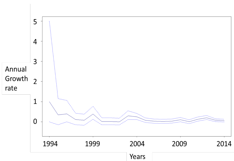
FIGURE 16 TAUX DE CROISSANCE* GÉOGRAPHIQUE — NOMBRE DE SITES NOUVELLEMENT OCCUPÉS DIVISÉ PAR LE NOMBRE DE SITES OCCUPÉS L'ANNÉE PRÉCÉDENTE) DE 1994 À 2014. APRÈS UNE PHASE DE DÉCROISSANCE DE LA VITESSE DE COLONISATION JUSQU'À LA FIN DES ANNÉES 90, LA PROGRESSION DE L'AIRE DISTRIBUTION DU LOUP RESTE DEPUIS RELATIVEMENT CONSTANTE. TIRE DE LOUVRIER ET AL. (2017).
