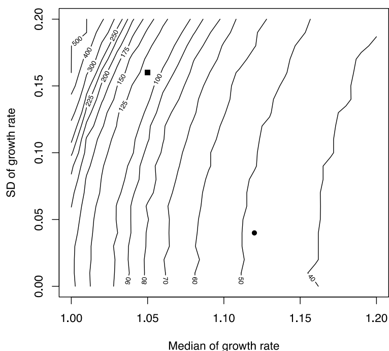
FIGURE 12 COURBES DE NIVEAUX DES SEUILS MINIMUM DE POPULATION Viable EN FONCTION DU TAUX DE CROISSANCE* DE LA POPULATION ET DE SA VARIANCE OBSERVEE. LE POINT NOIR REPRESENTE LE TAUX DE CROISSANCE* DE LA POPULATION FRANÇAISE ESTIME AVEC UN MODELE EXPONENTIEL, ALORS QUE LE CARRE NOIR REPRESENTE LE TAUX DE CROISSANCE* DE LA POPULATION FRANÇAISE ESTIME AVEC UN MODELE A CROISSANCE FREINEE. LA TAILLE MINIMALE DE POPULATION DEMOGRAPHIQUEMENT Viable EST ESTIMEE EN EXECUTANT 10 000 SIMULATIONS MONTE-CARLO SUR LA BASE D'UN TAUX DE CROISSANCE* TIRE D'UNE DISTRIBUTION NORMALE (A L'EXCLUSION DES VALEURS NEGATIVES, SOIT \lambda > 0 ). SE REPORTER A CHAPRON ET AL. (2012) POUR LES DETAILS.
