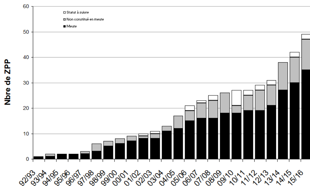
FIGURE 6 CINETIQUE DU NOMBRE DE ZONES DE PRESENCE DITE PERMANENTE DES LOUPS EN FRANCE DEPUIS 1992. SOURCE : RESEAU LOUP/LYNX, 2016.
