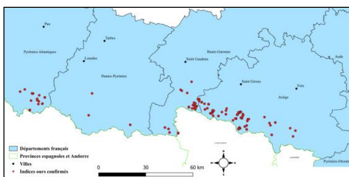
Répartition des indices d'ours « confirmés », relevés entre septembre et novembre 2025, dans les Pyrénées françaises.
